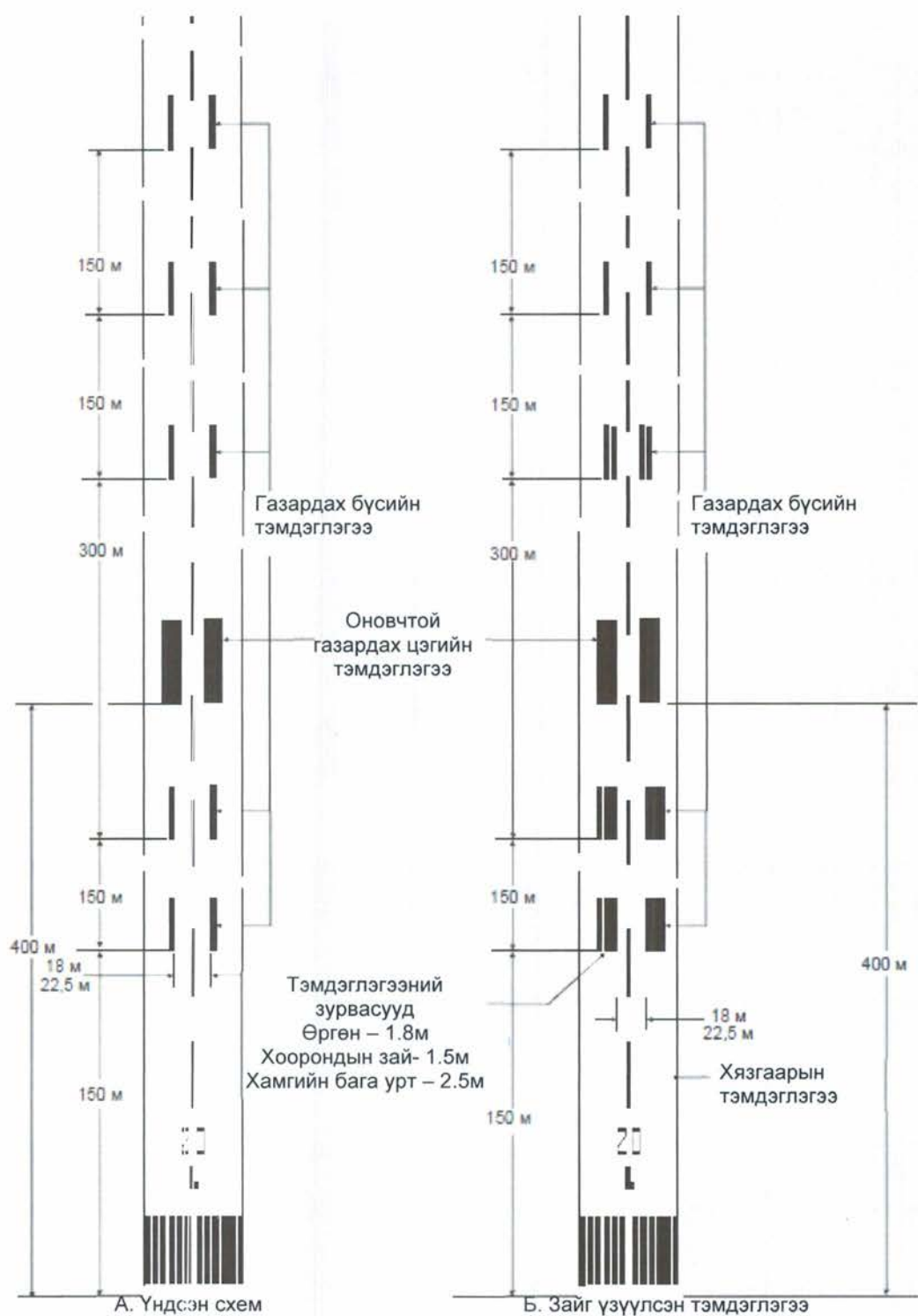
Зураг 5-5. Оновчтой газардах цэгийн болон газардах бүсийн тэмдэглэгээ (2400 м буюу түүнээс дээш урттай ХБЗ-ын хувьд)
