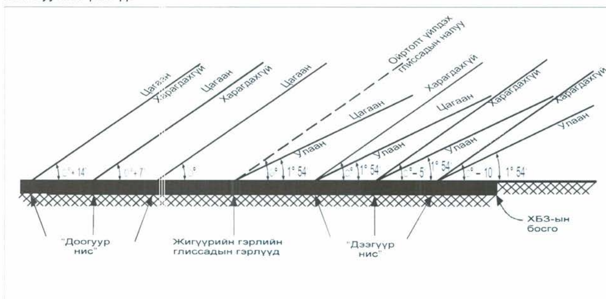
Зураг 5-18. T-VASIS ба AT-VASIS системийн гэрлийн цацраг ба өнцгийн тохируулга
