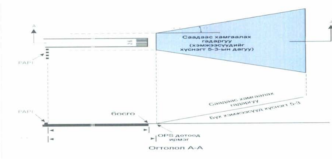
Зураг 5-21. Ил харааны налуууг заагч системийн саадаас хамгаалах гадаргуу
