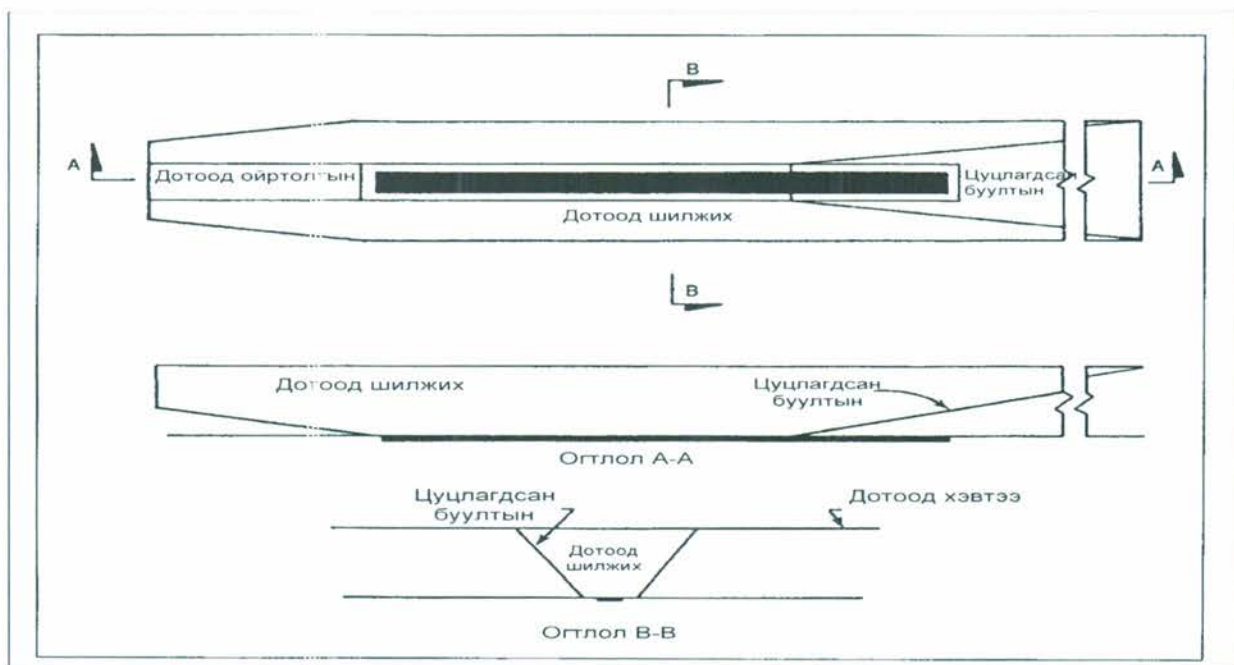
Зураг 4-2. Саадыг хязгаарлах гадаргуунууд: дотоод ойртолтын гадаргуу, дотоод шилжих гадаргуу ба цуцлагдсан буултын гадаргуу
