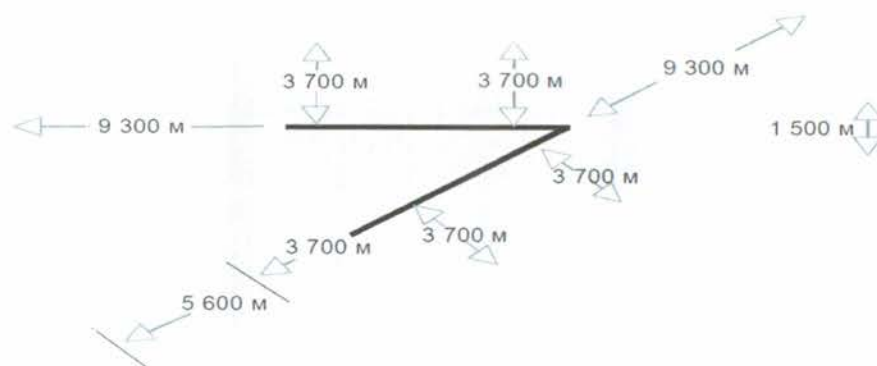
Зураг 5-12. Хэд хэдэн ХБЗ-тай үед лазерын цацрагийн нөлөөлөлгүй нислэгийн зурвас
