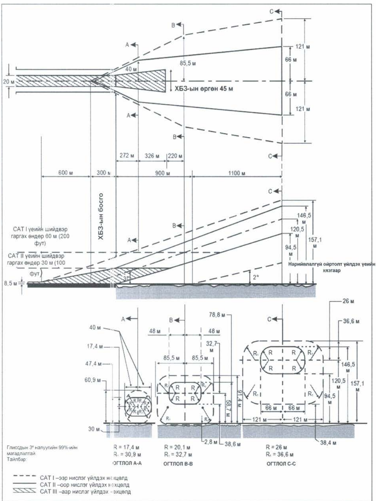
Зураг А-6. Нарийвчлалтай ойртолтын I, II ба III зэрэглэлтэй нөхцөлд гэрэл дохиоллыг төлөвлөх үеийн нислэгийн траекторийн диапозонууд
