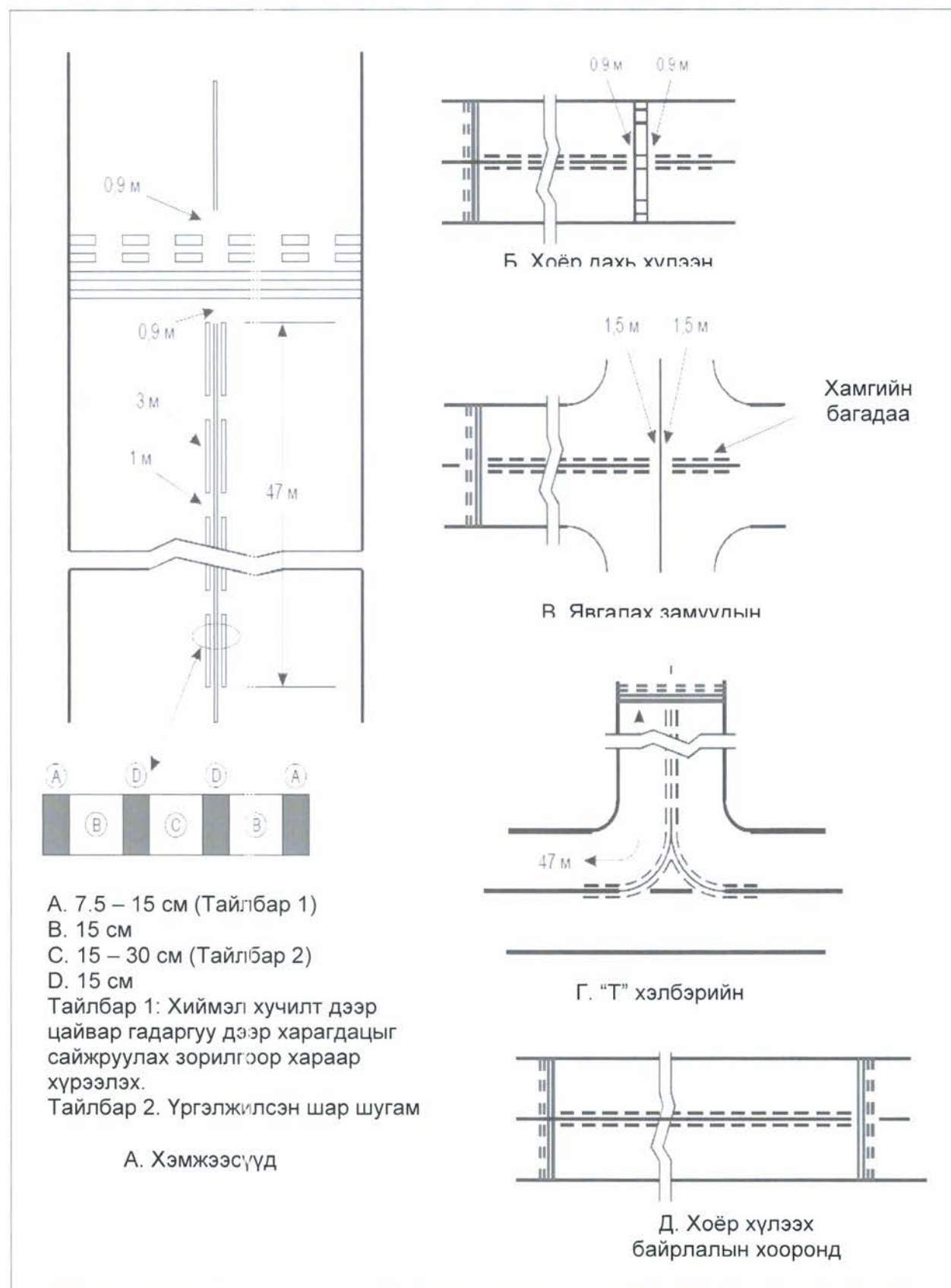
Зураг 5-7. ЯЗ-ын сайжруулсан тэнхлэгийн тэмдэглэгээ
