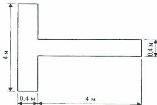
Зураг 5-16. Буултын чиглэл заагч тэмдэгт
