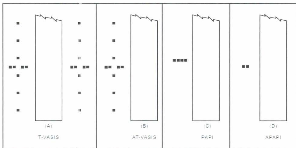
Зураг 5-16. Ил харааны ойртолтын налууг заагч систем
