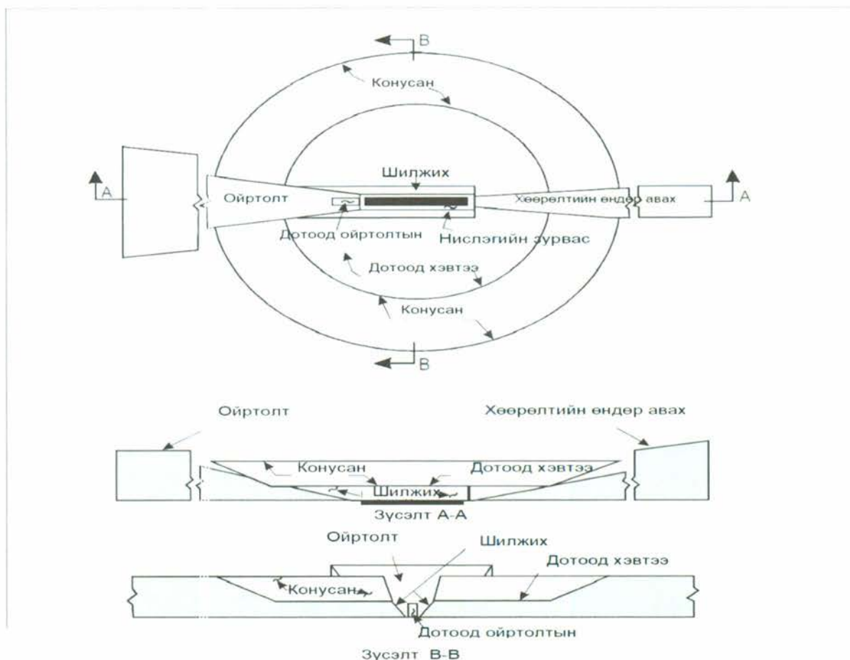
Зураг 4-1. Саадыг хязгаарлах гадаргуу
